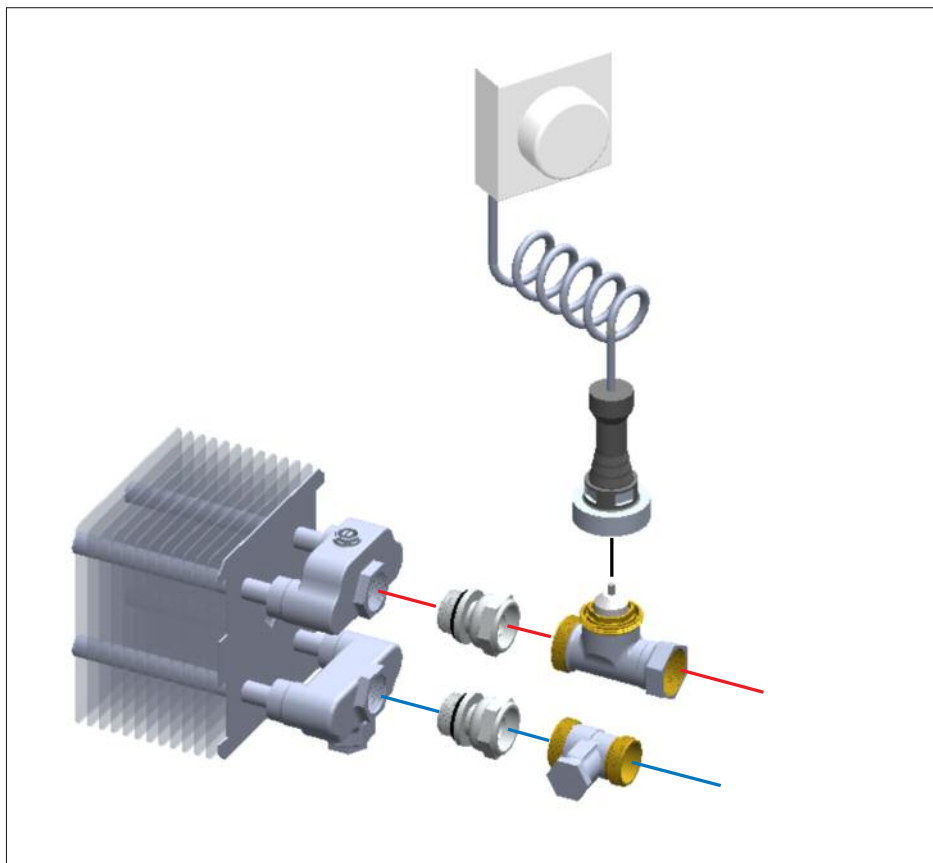
Anslutning längs med vägg
