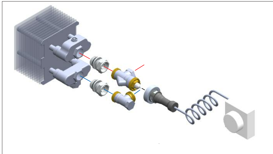
Anslutning ut från vägg
