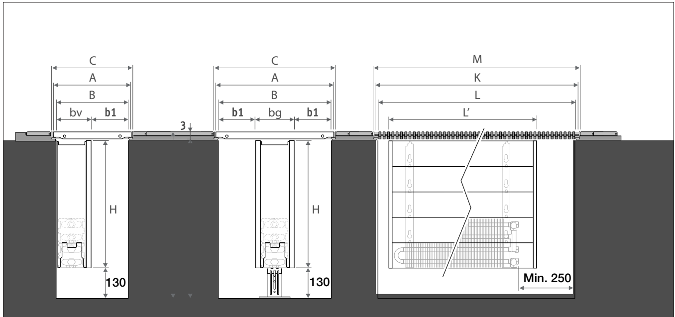
Bredder för Bygglin i golv
