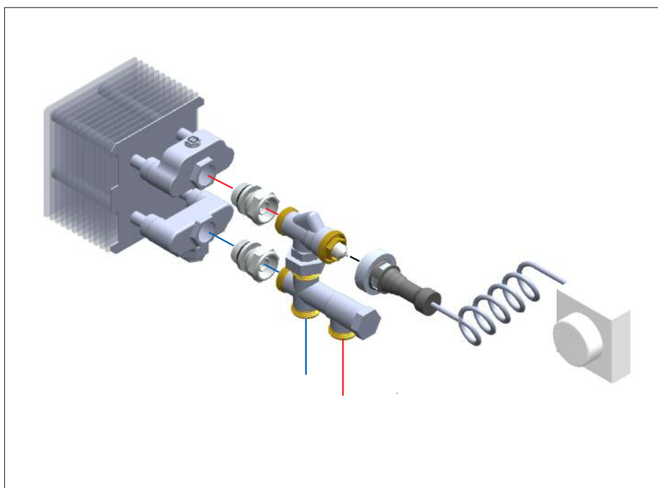
Anslutning med MMA-koppel.
