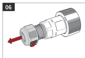
Løsne svivelen på den andre siden av kontakten.
