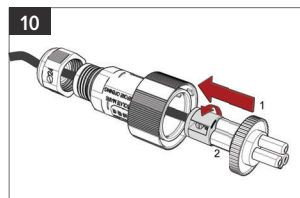
Skyv kjernen inn i huset. Og stram den.
