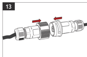
Sett de to delene sammen
