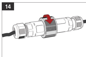
Stram til koblingen mellom de to husene
