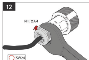
Stram svivelen til 2,4/4 Nm.
