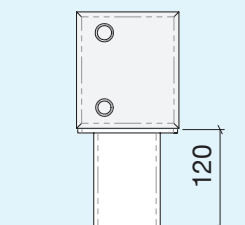
1. Gulvkonsoll C-profil
