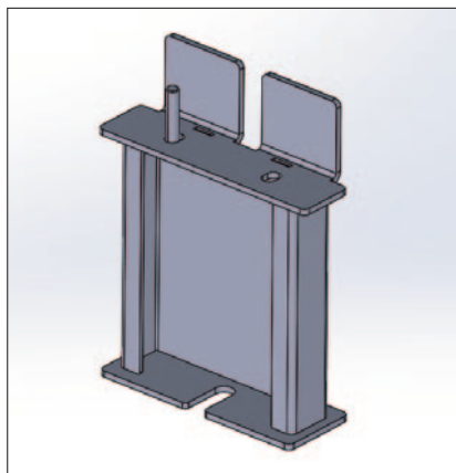
KONSOLLTYPE 1, C-KONSOLL
