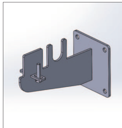
KONSOLLTYPE 3, VEGGBRAKETT
