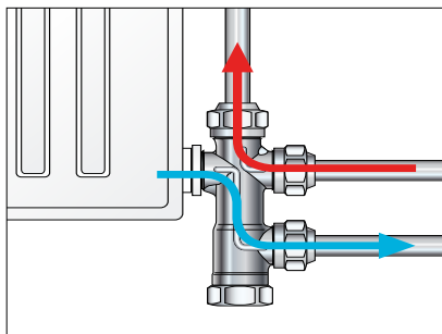
Sidoanslutning
