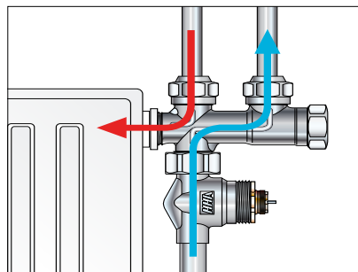
Toppanslutning
