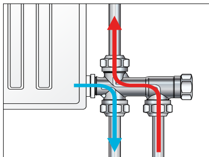
Bottenanslutning
