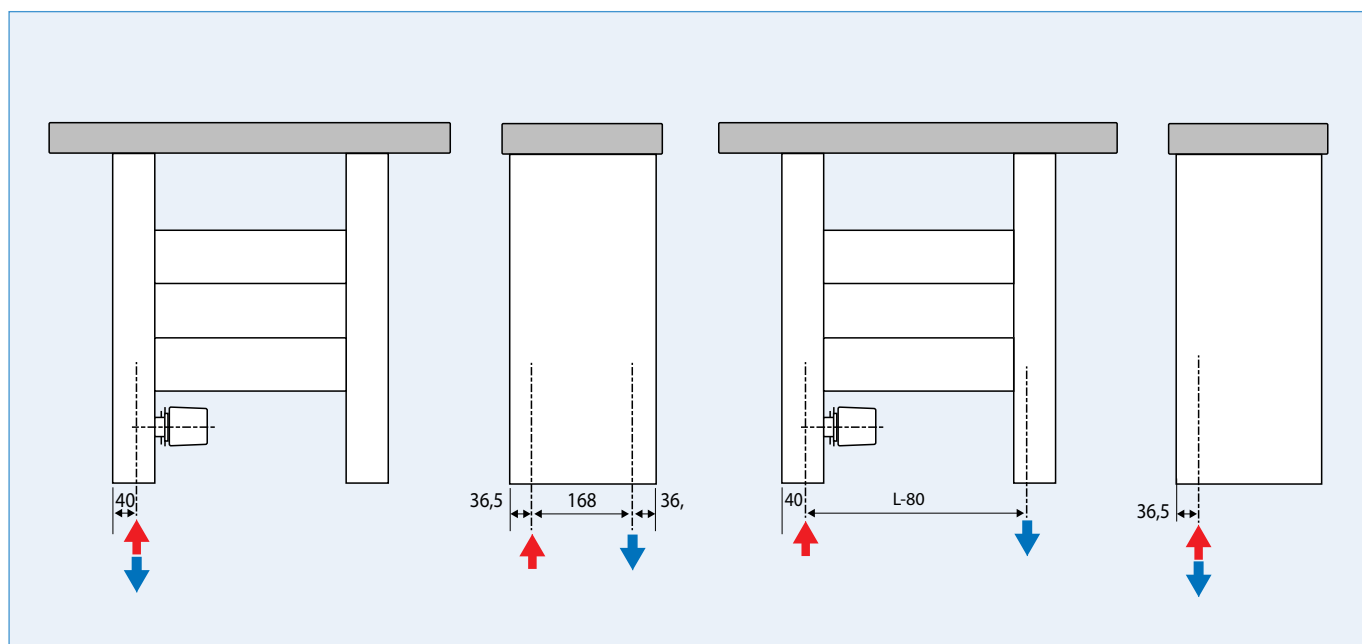
Type 50/54. Venstre. Tilkoblingsalternativ 1 Høyre. Tilkoblingsalternativ 2
