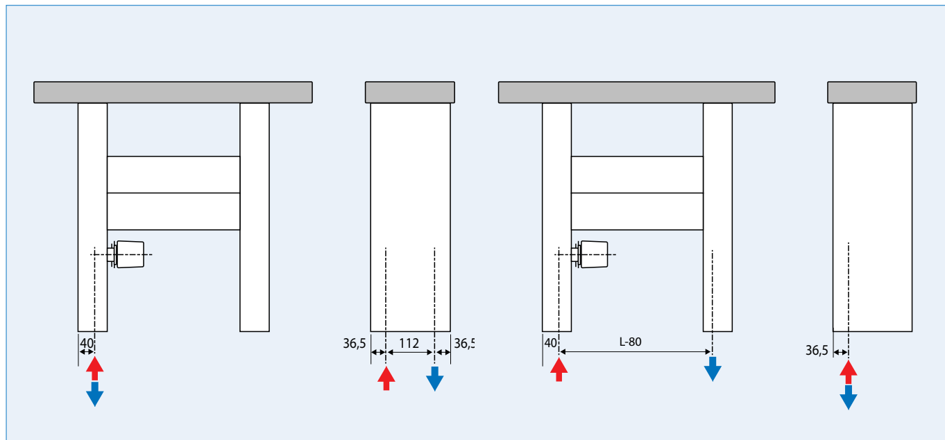
Type 43/43. Venstre. Tilkoblingsalternativ 1 Høyre. Tilkoblingsalternativ 2
