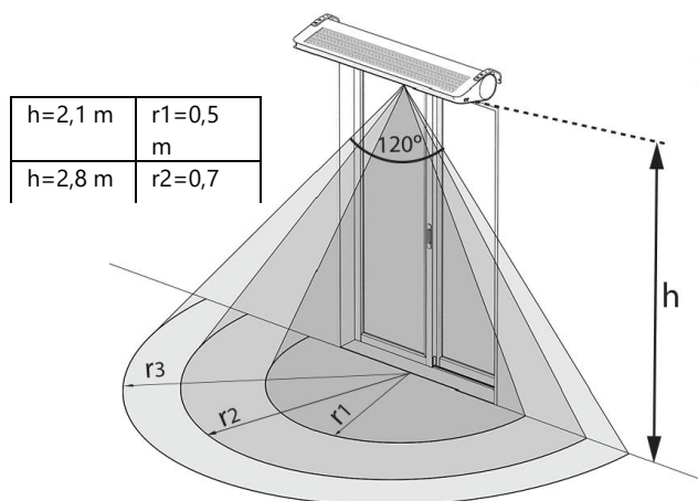
RYS. 12.3 OBSZARU ZADZIAŁANIA CZUJNIKA RUCHU.
