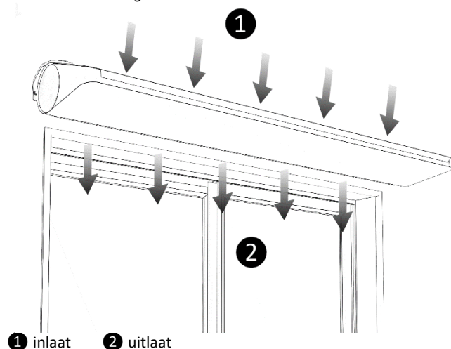
AFB. 2.1 RICHING LUCHTSTROOM.
