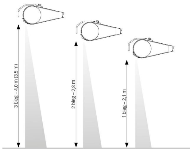
RYS. 2.2 ZASIĘG POWIETRZA NA POSZCZEGÓLNYCH BIEGACH.
