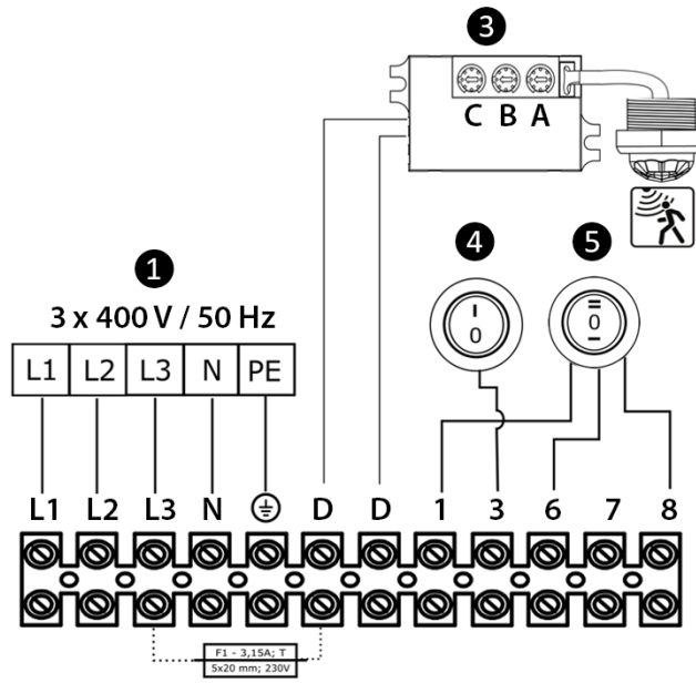
СХЕМА 13.2 ПИТАНИЕ 3N ~ 400В/50Гц
