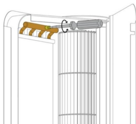
RYS. 17.2. WBUDOWANY ZAWÓR ODPOWIEZRZAJĄCY.
