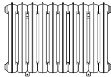
560 x 852 10 seksjoner
