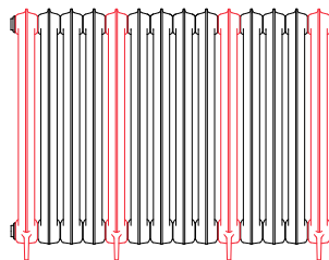
920 x 1180 14 seksjoner (4+10)
