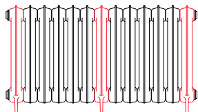
620 x 1098 13 seksjoner (3+10)
